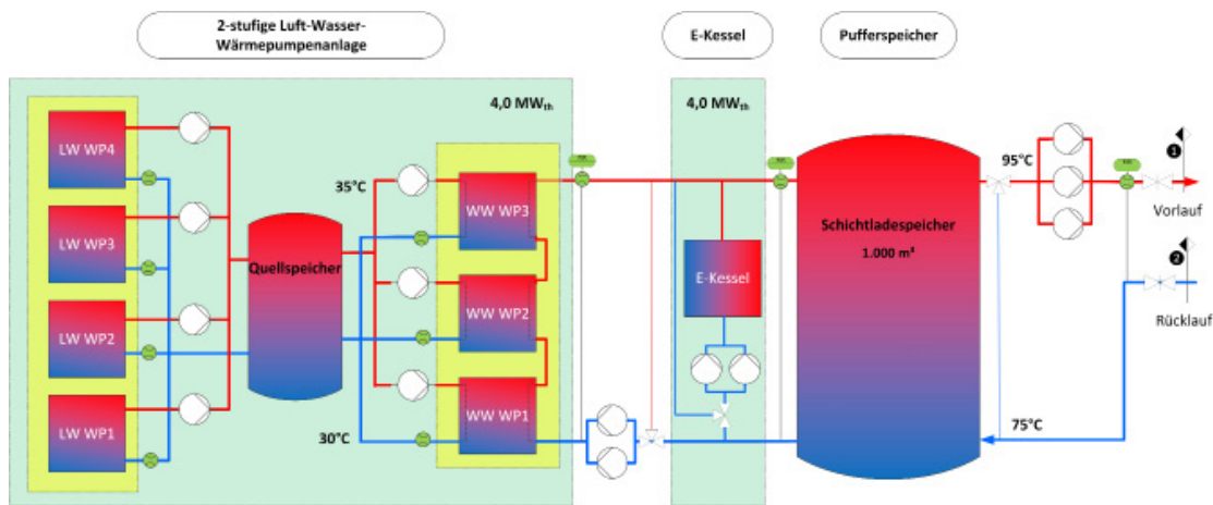
Visualisierung Anlagenfließschema des Leuchtturmprojektes Power-to-Heat-Anlage (2-stufige Wärmepumpe, E-Kessel und Pufferspeicher).
